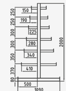
Langgutregal doppelt
