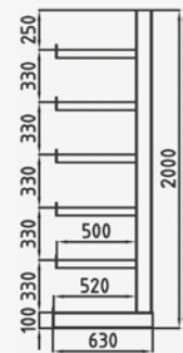
Kragarmregal einfach
