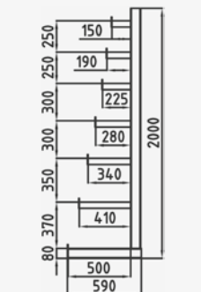
Langgutregal einfach
