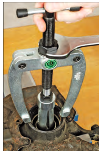
Komplette Abziehvorrichtung, bestehend aus Innenauszieher Nr. 21 und Gegenstütze Nr. 22
